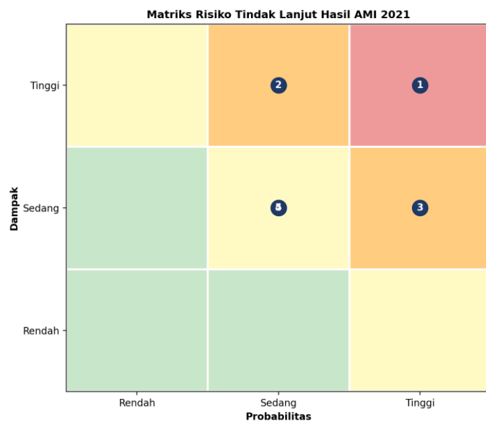
Grafik 5.2 Peta Matriks Risiko (Probabilitas x Dampak), AMI 2021
